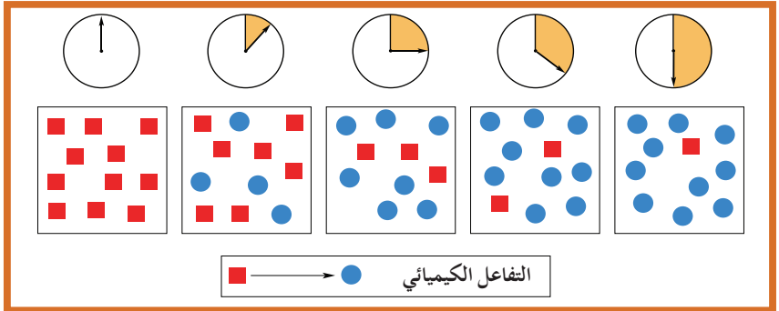
شكل (33) مع مرور الوقت ، تتناقص كمية المتفاعلات (المرتعات الحمراء) وتزداد كمية النواتج (الدوائر الزرقاء).
