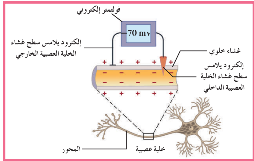
(شكل 14) يشير الفولتметр الإلكتروني إلى وجود فرق جهد لغشاء الخلية العصبية يعرف بجهد الراحة ويساوي -70\text{ mV} ، وذلك بسبب اختلاف الشحنات بين السطح الداخلي لغشاء الخلية (وهو سالب) والسطح الخارجي لغشاء الخلية (وهو موجب).
