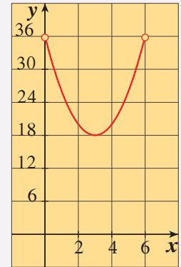
شكل (1) بيان الدالة S
